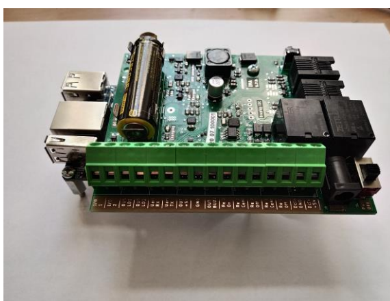
Řídící elektronika pro komunikaci GVM.01 – vydavač golfových míčků – platební terminál - banka
